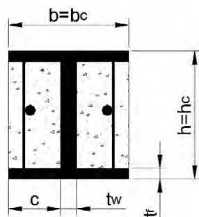
Fig. 7.6.1 - Rapporti dimensionali
